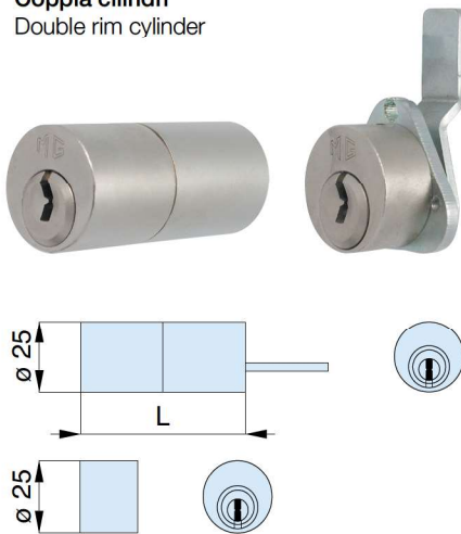
Coppia cilindri Double rim cylinder
