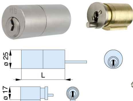
Coppia cilindri Double rim cylinder
